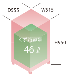
【本体サイズ】 W515×D555×H950mm (スイッチ含むH961mm)
